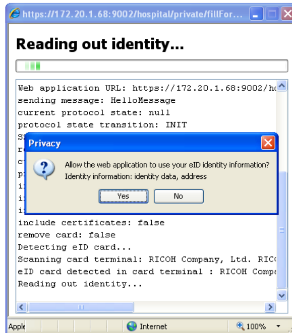
Figure 14 : Lecture carte d'identité
